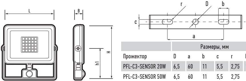
Рис. 1 Прожектор PFL-C3-SENSOR
