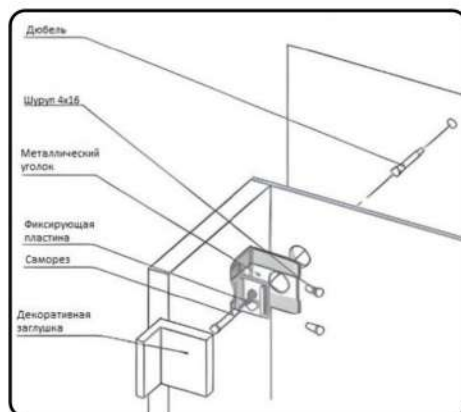
Крепление навеса шкафа
