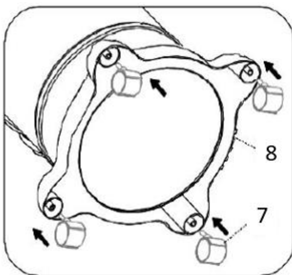
Сборка колес
