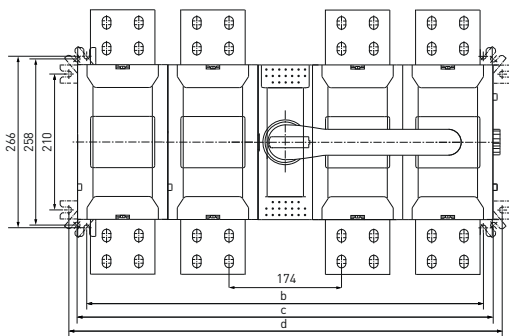
Рисунок 7а – Монтажные размеры рубильника PowerSwitch 4000 А
