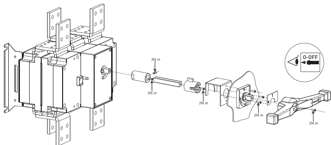
Рисунок 16а – Монтаж выносной ручки для рубильников 2000-2500 А
