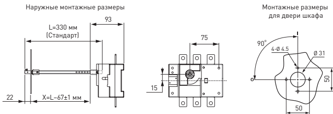
Рисунок 14б – Монтажные размеры при установке на дверцу шкафа для рубильников 160 А
