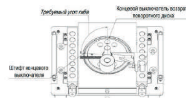
Рис. 6. Установка углагиба
