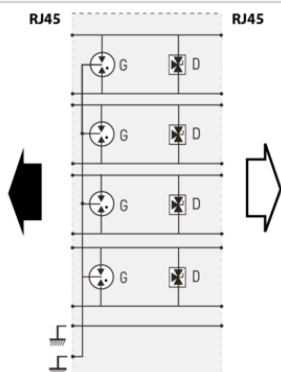
Р: 3-электродный GDT D: фиксирующий диод
