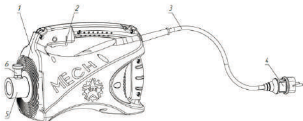
Рис. 1. Схема устройства универсального привода VPK MECH: 1 – корпус в сборе, 2 – клавиша включения, 3 – кабель, 4 – вилка кабельная 230 В/16 А с заземляющим контактом, 5 – разъем для подключения гибкого вала с вибронаконечником, 6 – пружинный фиксатор
