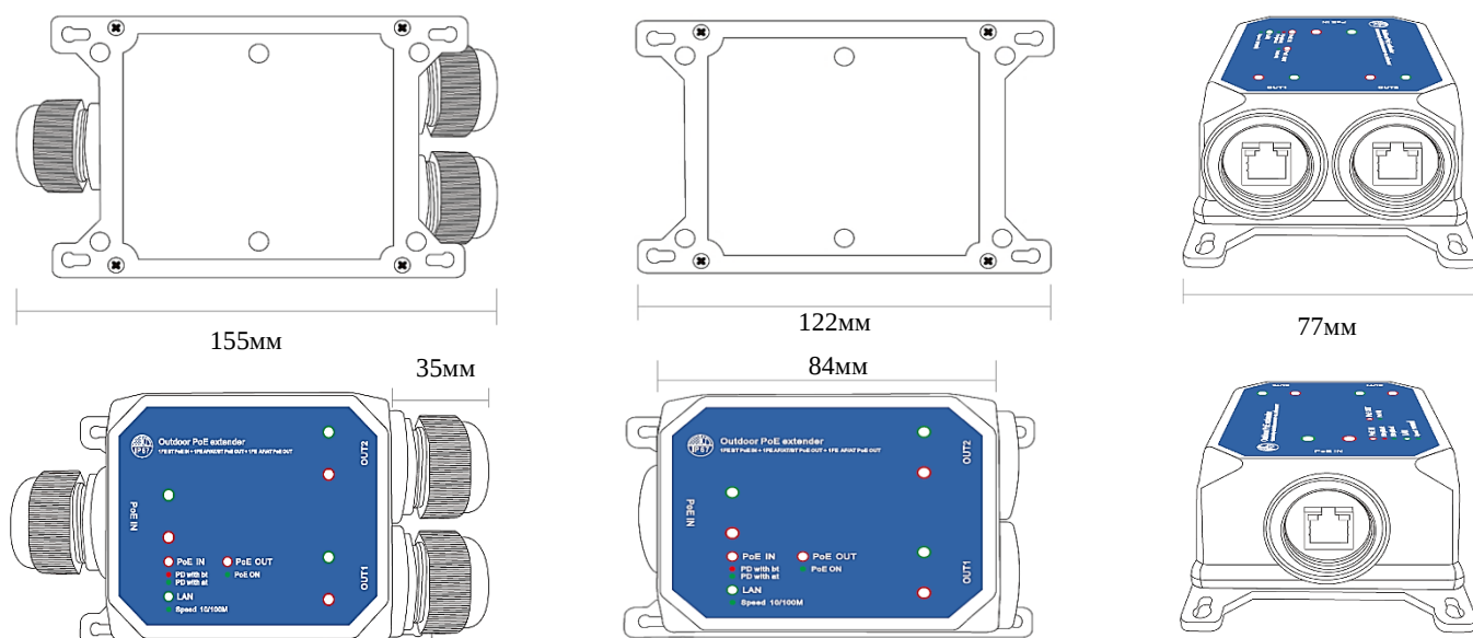
Рис. 1. Габаритные размеры
