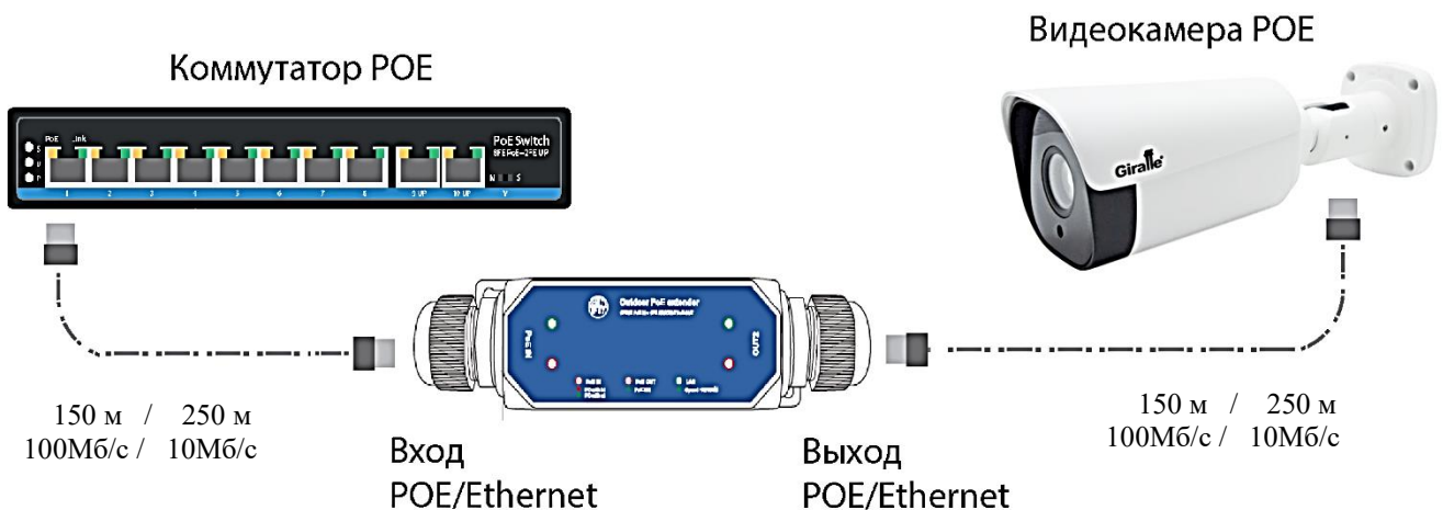
Рис. 4. Подключение устройств к Изделию
