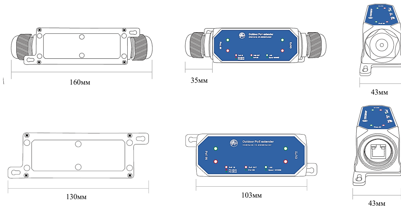
Рис. 1. Габаритные размеры
