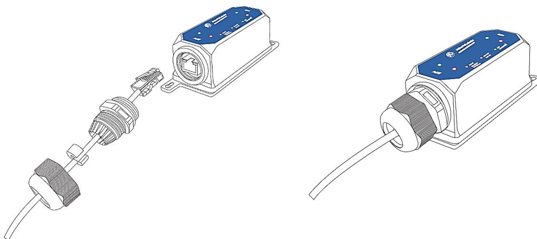
Рис. 3. Подсоединение к Изделию
