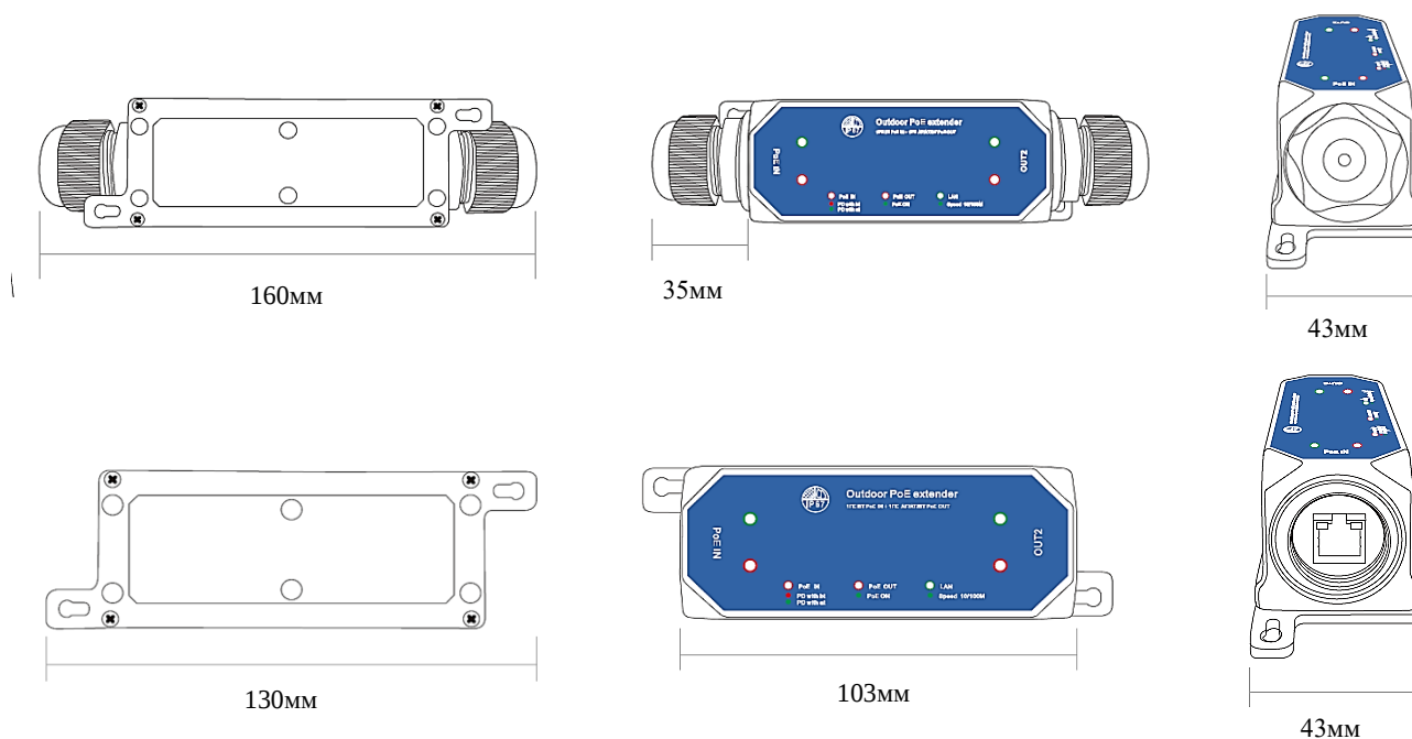
Рис. 1. Габаритные размеры
