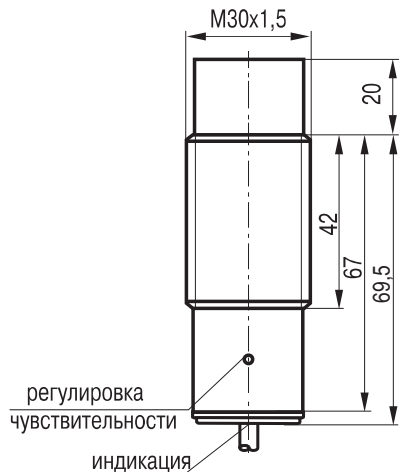
Габаритный чертеж
