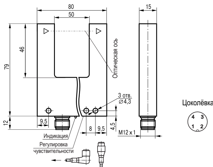
Габаритный чертеж
