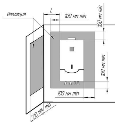
Рис. Установка аппарата на трудносгораемых стенах.
