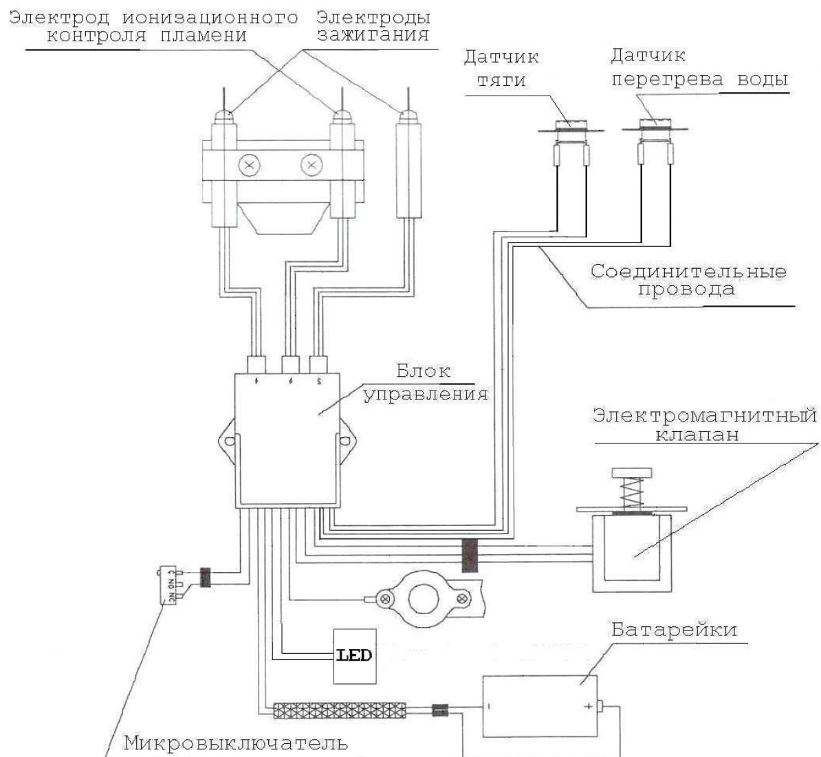
Рис. 2. Схема электрическая
