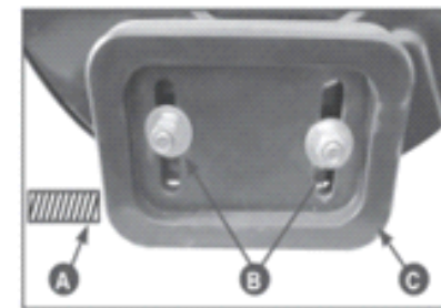
Рис. 9 Установка троса управления дефлектора жёлоба
