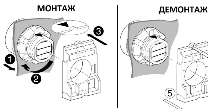
Рис.13 Монтаж и демонтаж выключателя пластикового.
