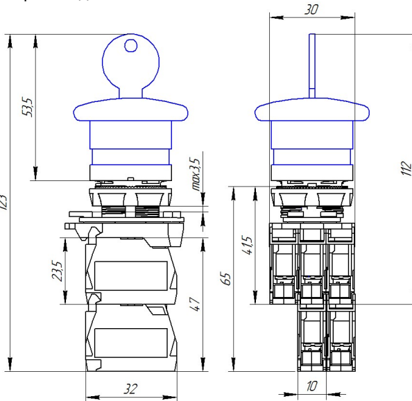
Рис.5. Выключатель кнопочный с фиксацией (возврат ключом).
