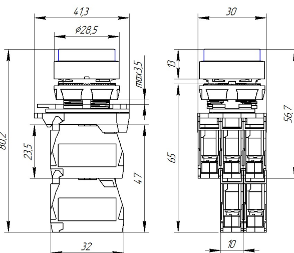
Рис.7. Выключатель кнопочный с выступающим цилиндрическим толкателем.
