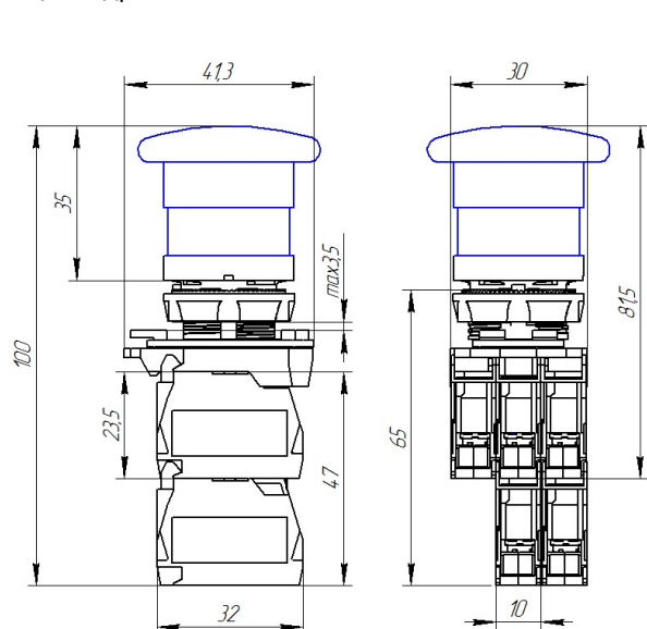
Рис.4. Выключатель кнопочный с фиксацией.
