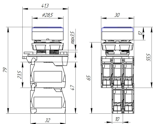
Рис.6. Выключатель кнопочный с подсветкой.
