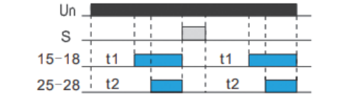
Рисунок 3.2 – Функциональная диаграмма работы реле
