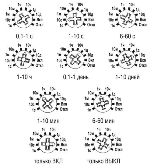
Рисунок 3.3 – Диапазоны выдержки реле
