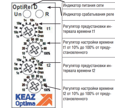
Рисунок 3.1 – Панель управления
