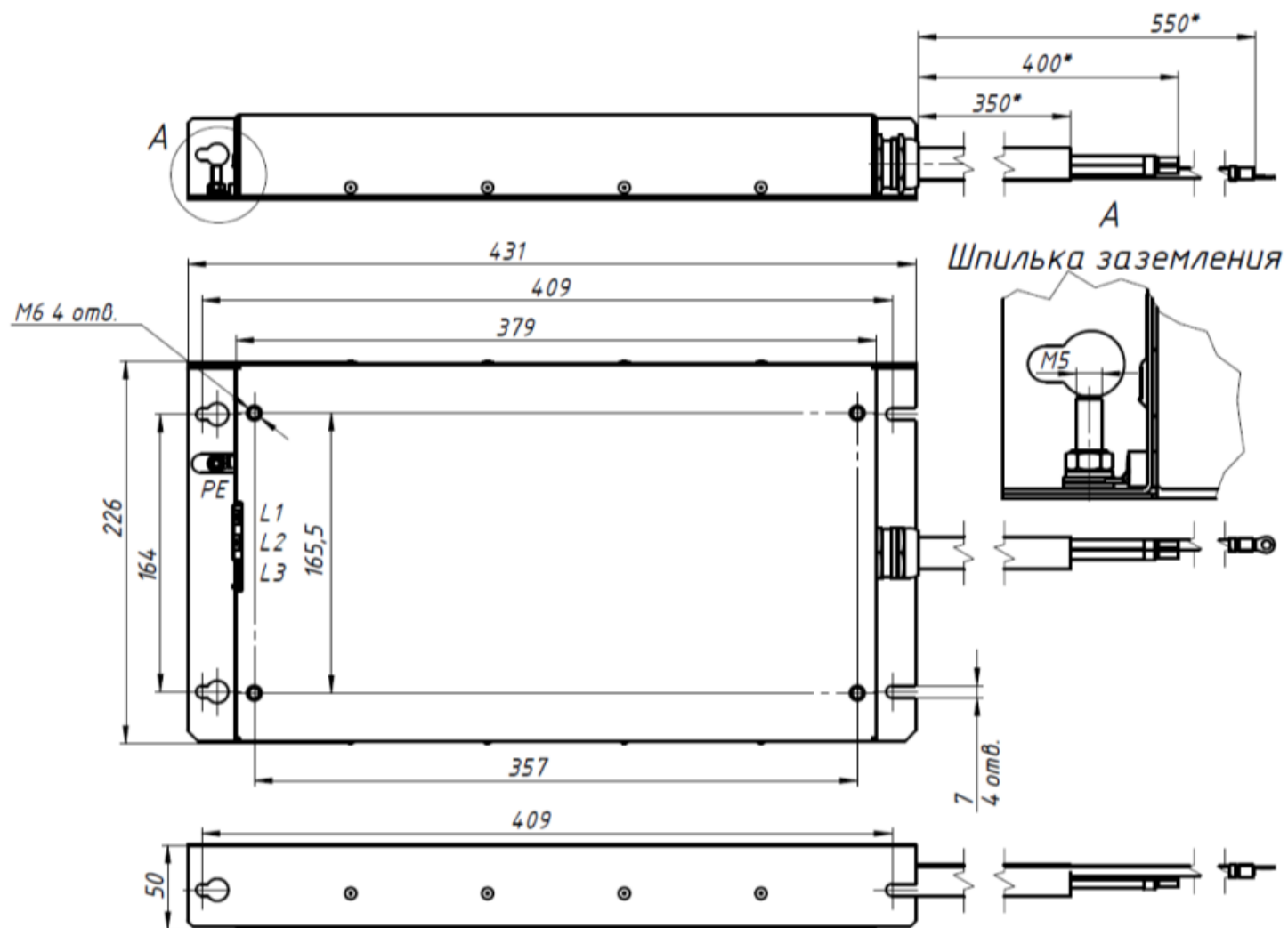
Размеры фильтров ФКРС-7,5-0,4-00 и ФКРС-11-0,4-00
