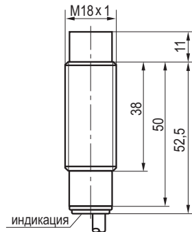
Габаритный чертеж
