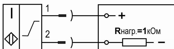
Схема подключения к оборудованию
