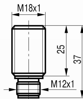
Габаритный чертеж
