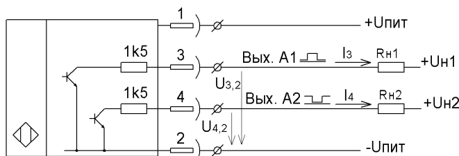
Схема подключения
