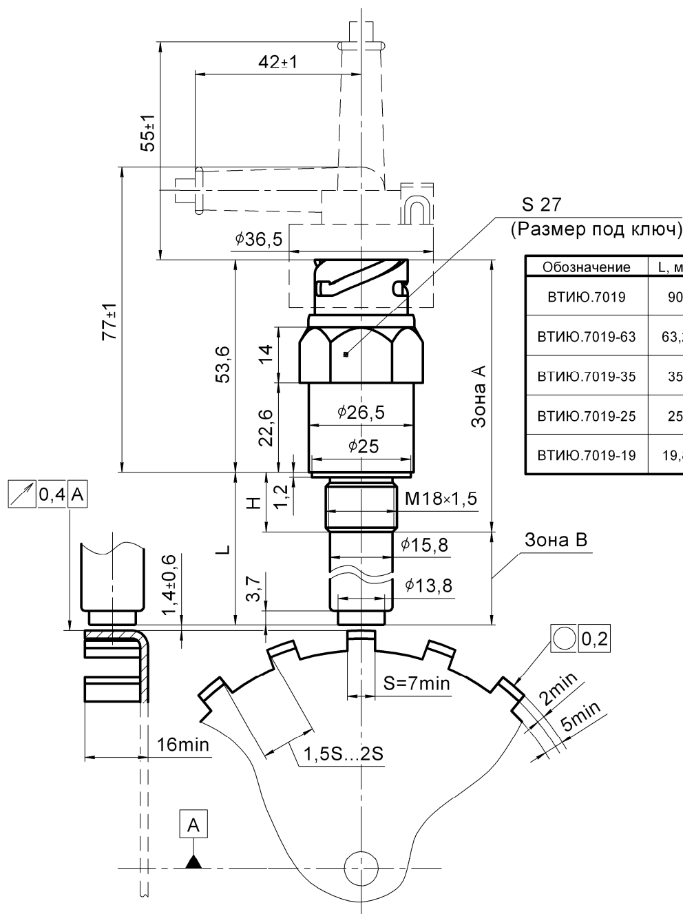
Габаритный чертеж
