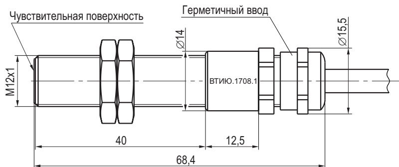
Габаритный чертеж
