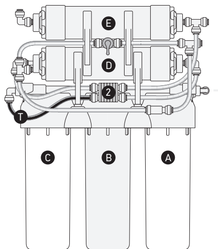
Рис.4. Схема подсоединения трубки (Т) к управляющему клапану (2).
