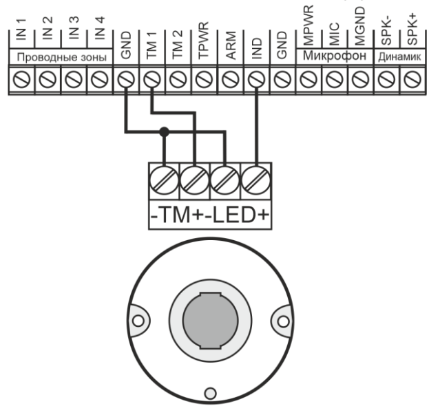
Клеммная колодка ИПРО - 7 (6)
