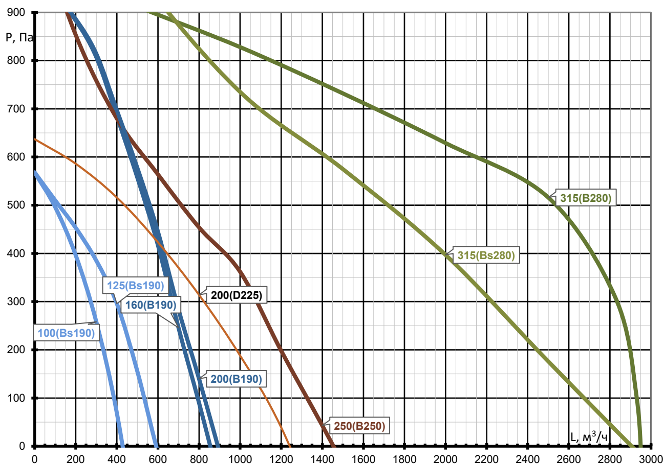
Аэродинамические характеристики
