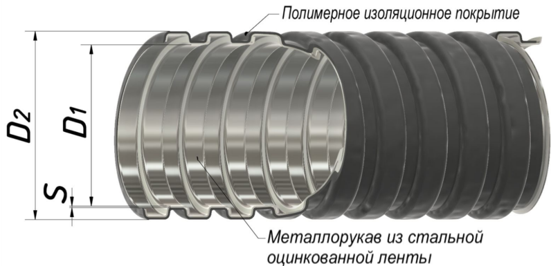
Рисунок 1. Металлорукав типа P3-ЦП нг черный
