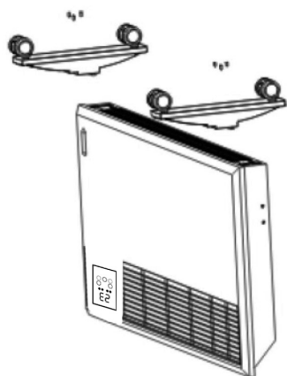
Рис. 3. Схема крепления стоек
