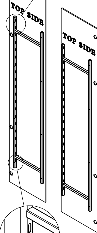
Верх рамы
