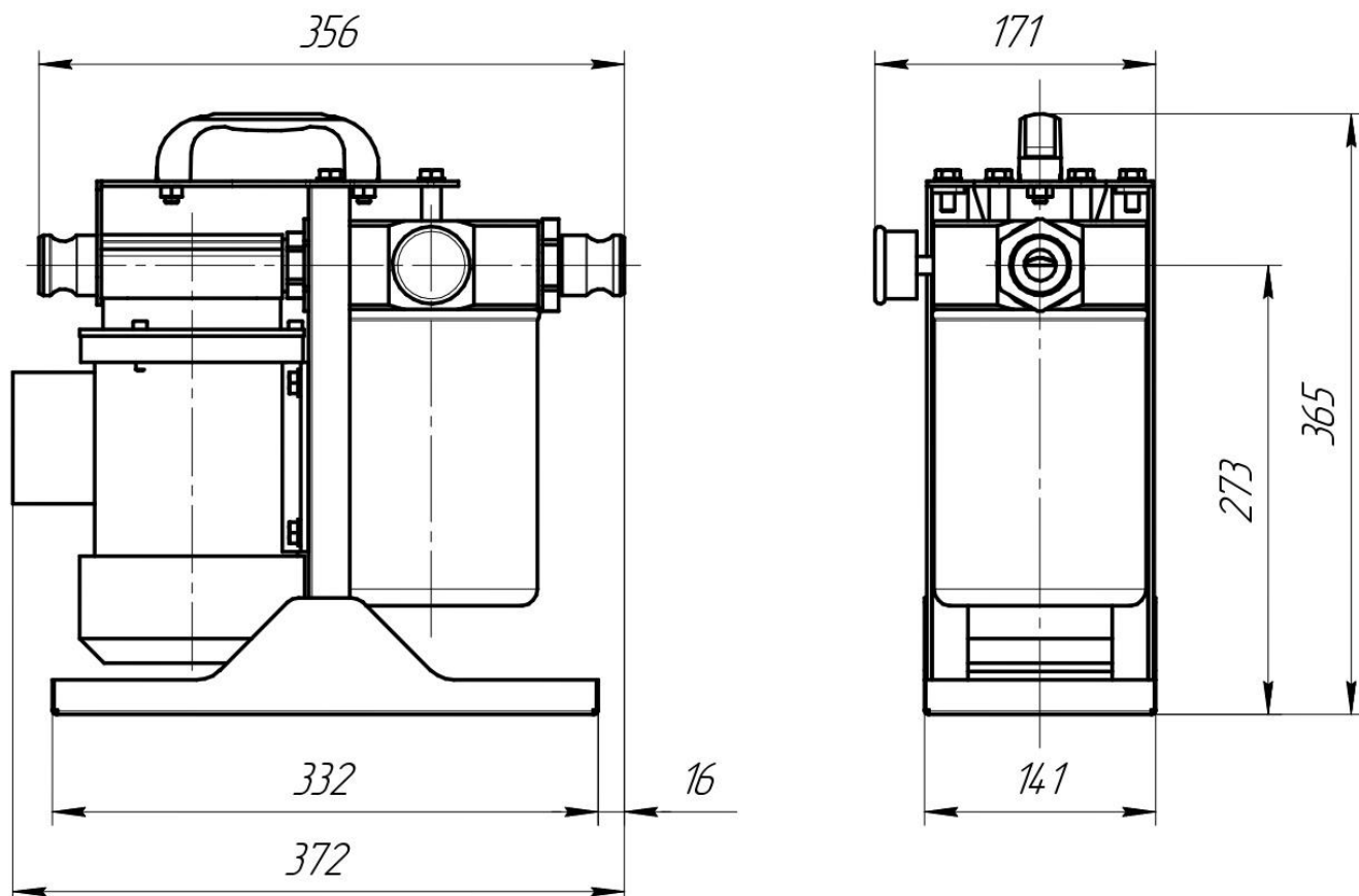
Габаритные размеры.
