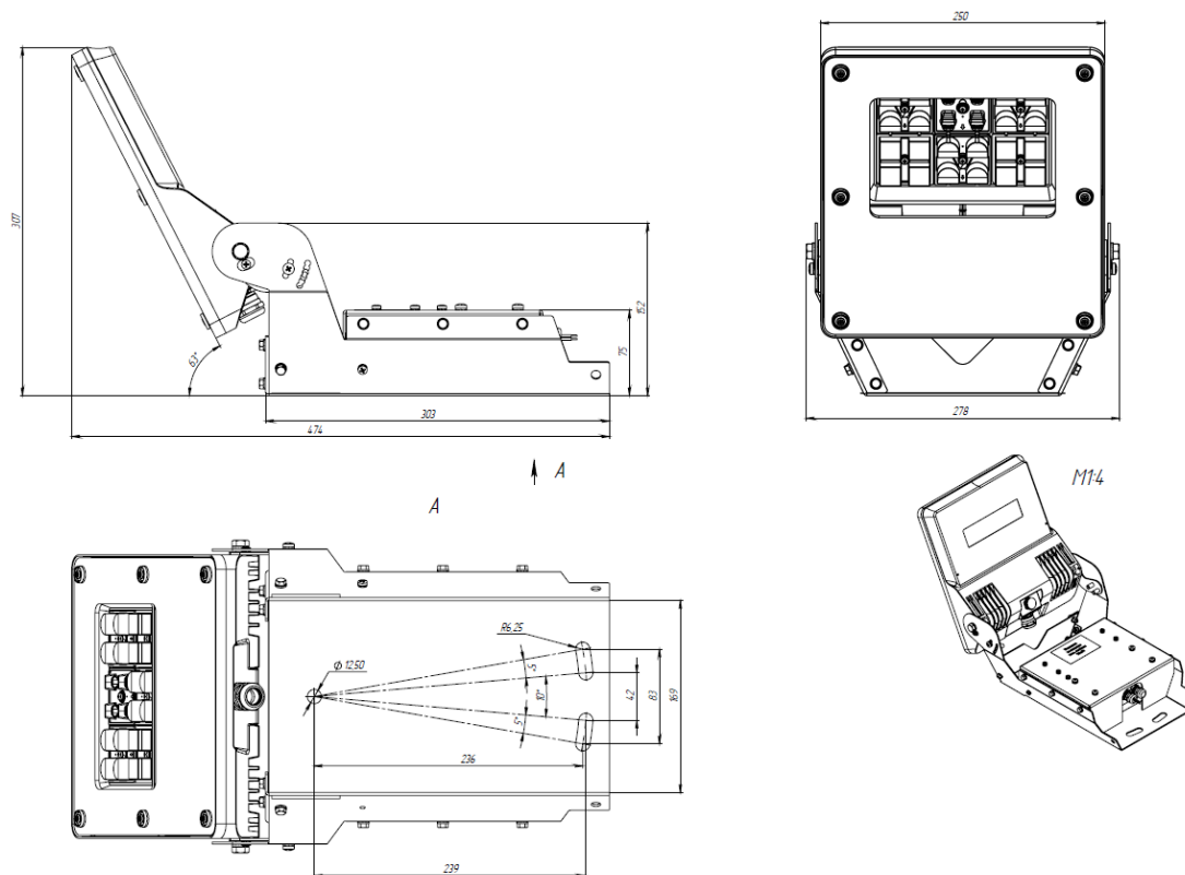
Габаритный чертёж светильников VA1853.00.000 60 Вт
