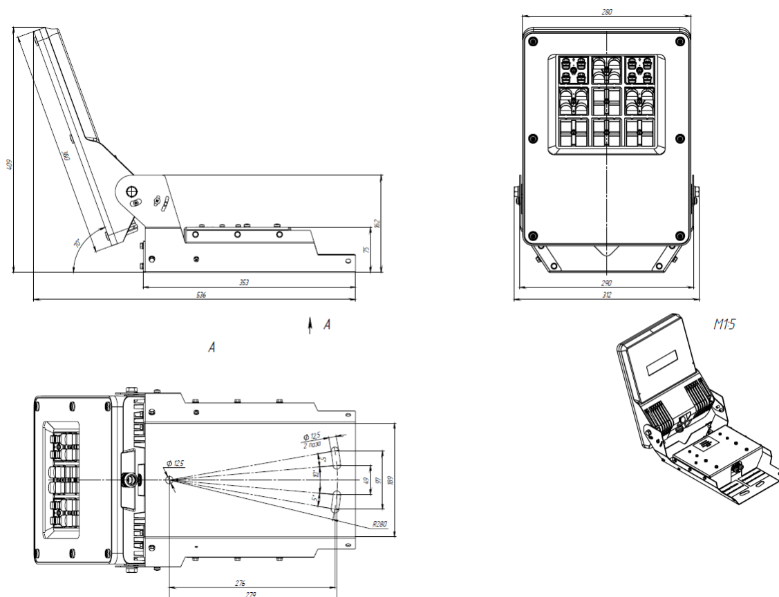
Габаритный чертёж светильников VA1854.00.000 80 Вт
