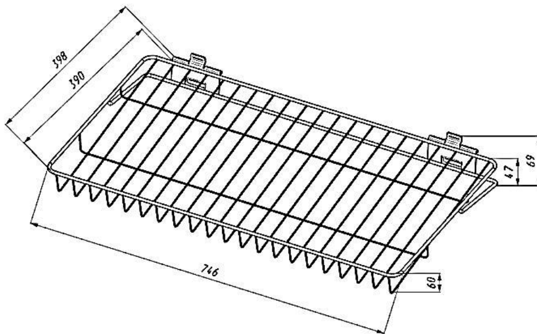
Рисунок 1 – Полка для обуви REL.01.0301.03. Общий вид и габаритные размеры, мм
