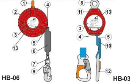
Рис. 1. Внешний вид, составные части и параметры
