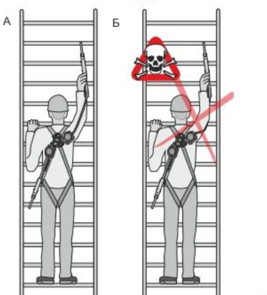
Рис. 11. Использование двухплечевого «НВ-02»
