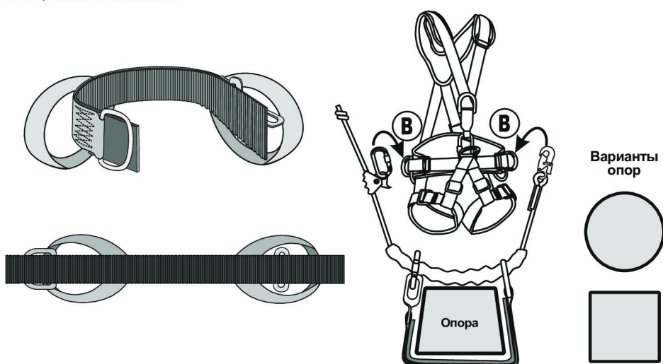
Рис. 5. Присоединение комплекта
