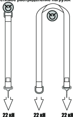
Рис. 5. Присоединение комплекта
