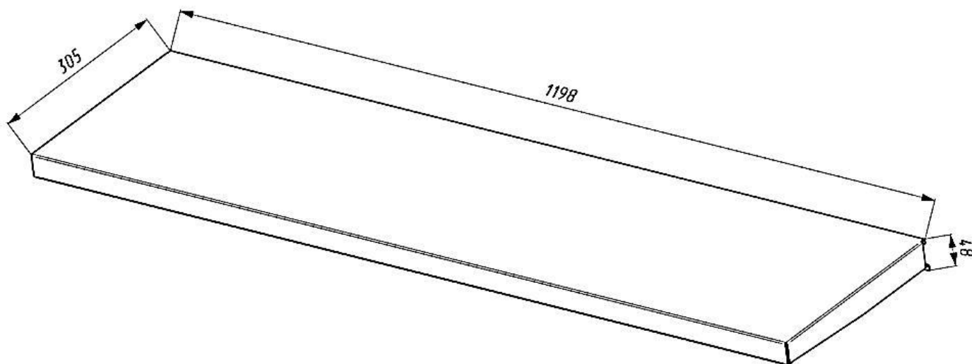
Рисунок 2 – Полка сплошная 1200 REL.01.0301.02. Общий вид и габаритные размеры, мм
