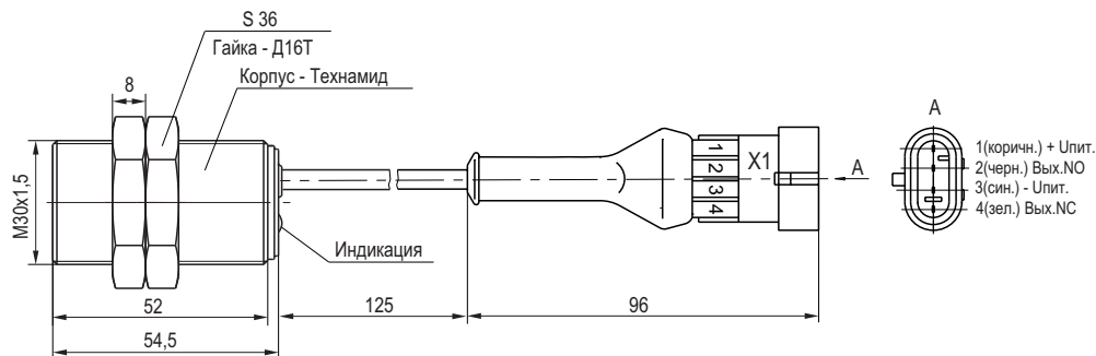
Габаритный чертеж
