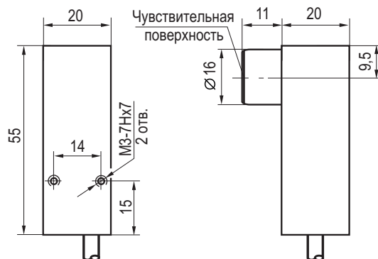
Габаритный чертеж
