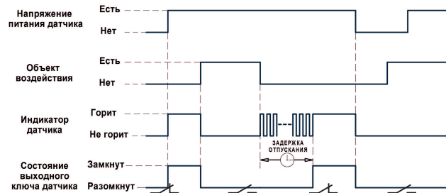
Диаграмма работы датчика
