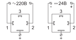
Схемы подключения катушки
