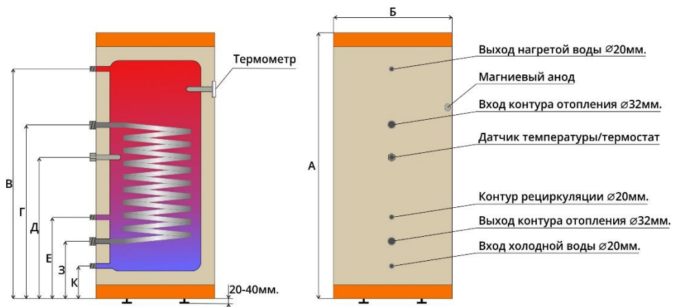
Рис 1. «Эрни 150»
