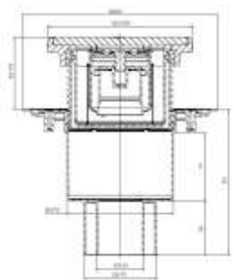
Трап HL310PrblueG
