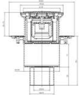
Трап HL310PrblueR
