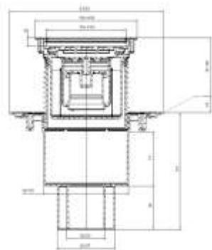
Трап HL310Prblue 3020
