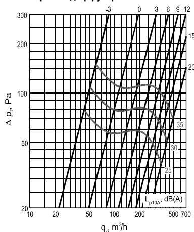
Открытие диффузора DVS-U 200 в мм
