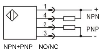
NPN+PNP NO/NC
