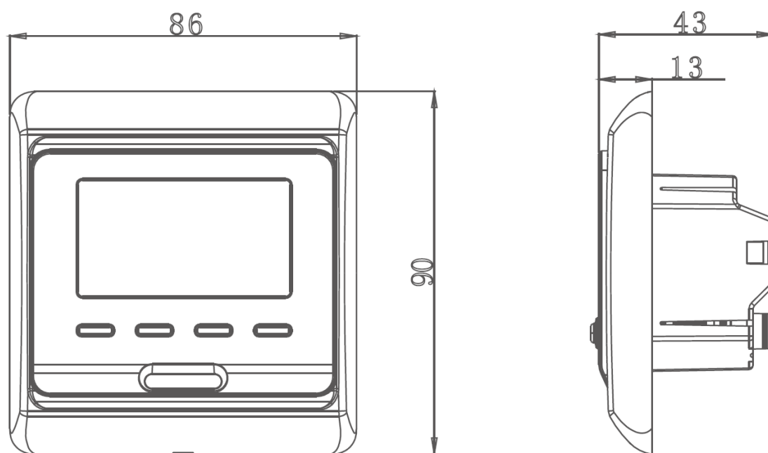
Рисунок – 2. Габариты
