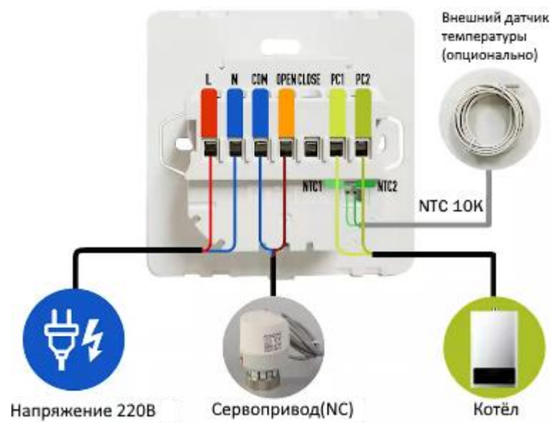
Рисунок – 3. Пример подключения №1
