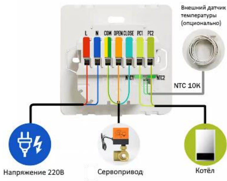
Рисунок – 3. Пример подключения №1
