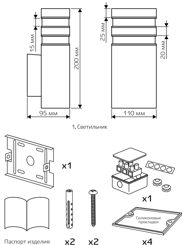
2. Монтажный комплект
