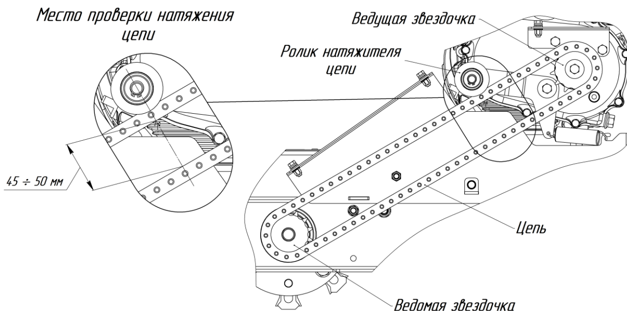
Рис.10. Проверка натяжения цепи.
