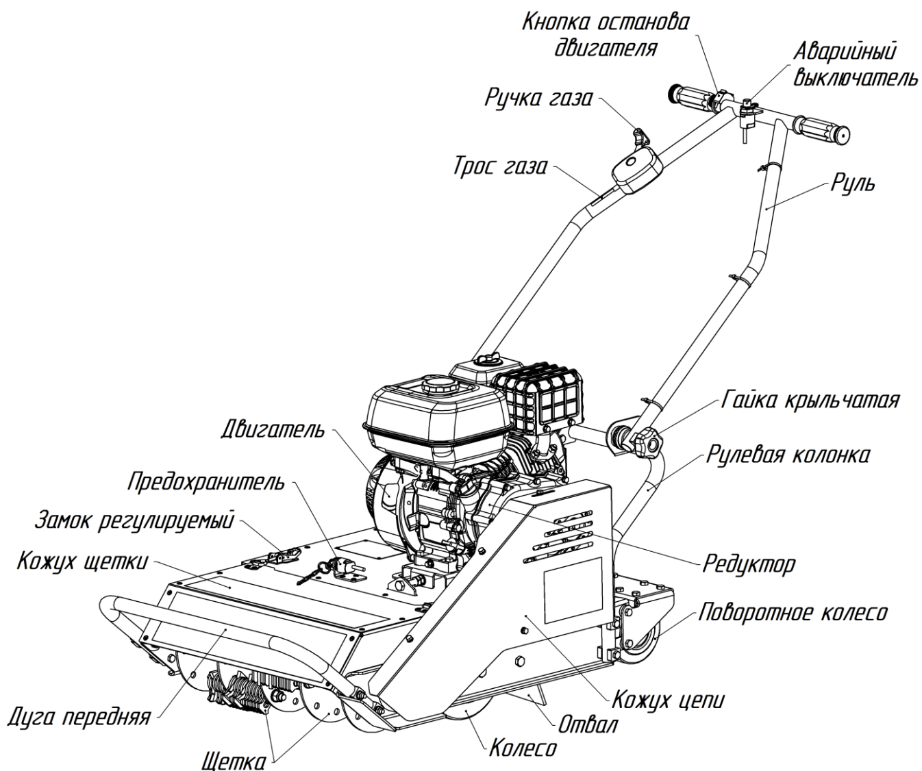
Рис.1. Общий вид ледокола ЛК1.
