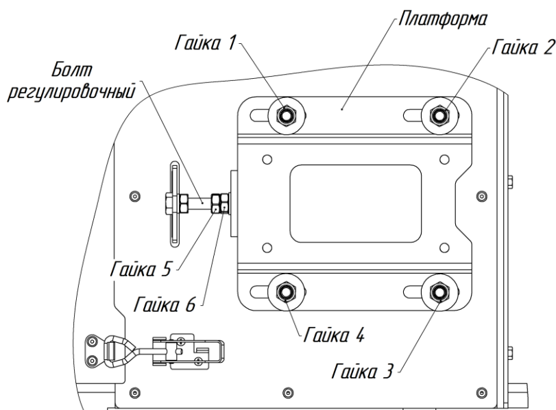
Рис.11. Схема натяжения цепи.
