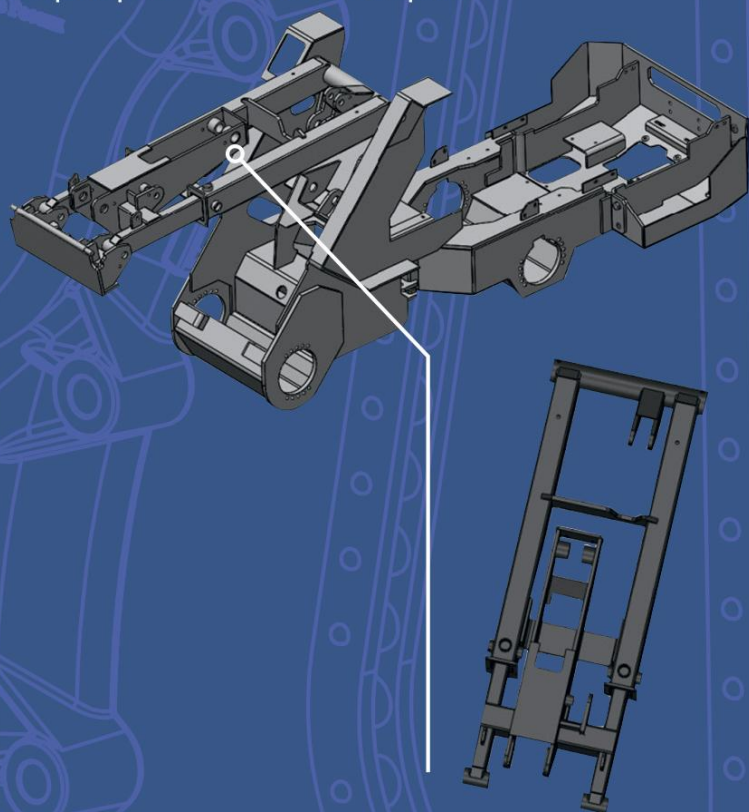
Шарнирно-сочлененная рама
