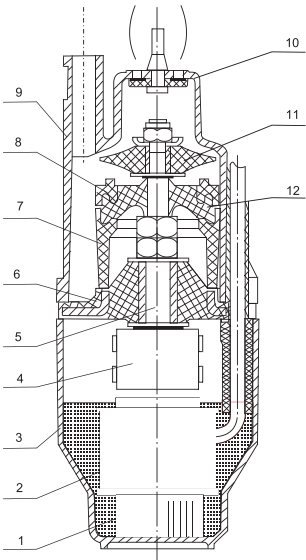
Рис. 1. Устройство насоса
