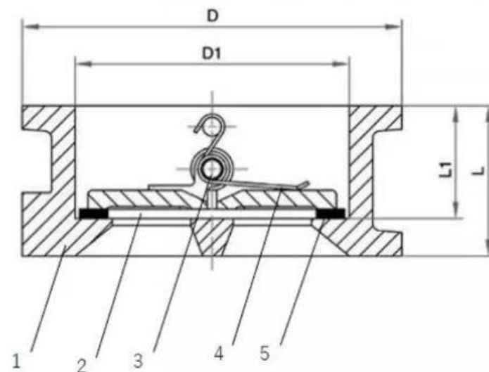
Эскиз клапана обратного чугунного двухдискового Сі Ду100 Ру16
