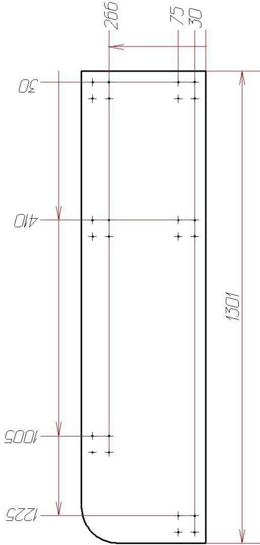
Поз. 8 Стенка горизонтальная
