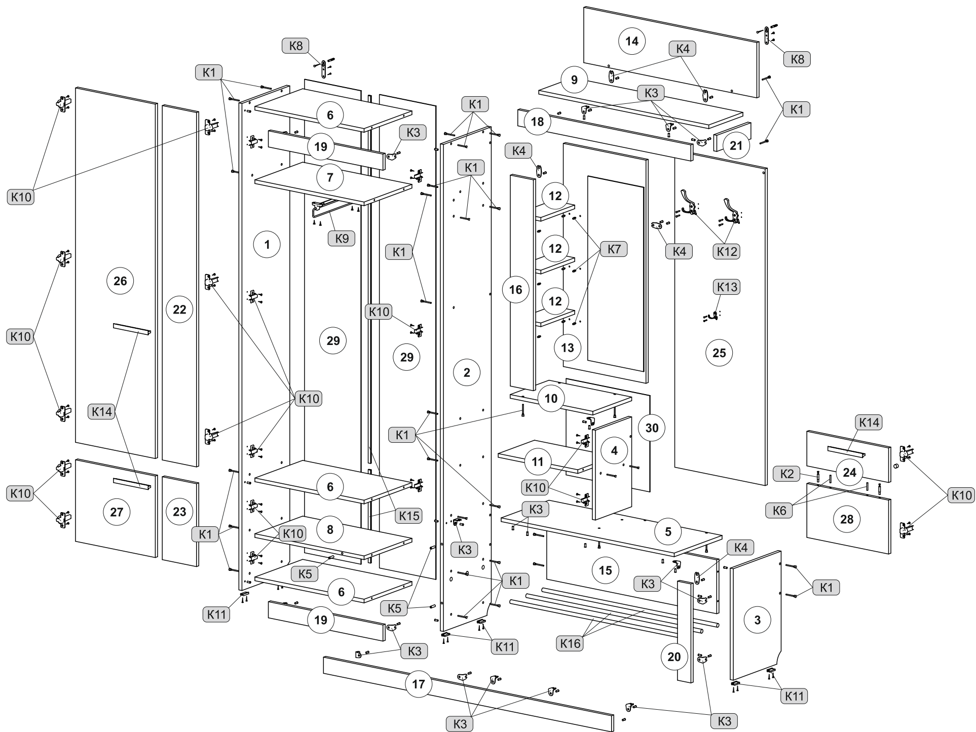
Схема 1. Сборка прихожей
