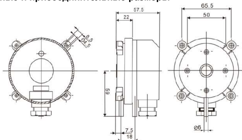
Рис.1. Габаритные и присоединительные размеры
